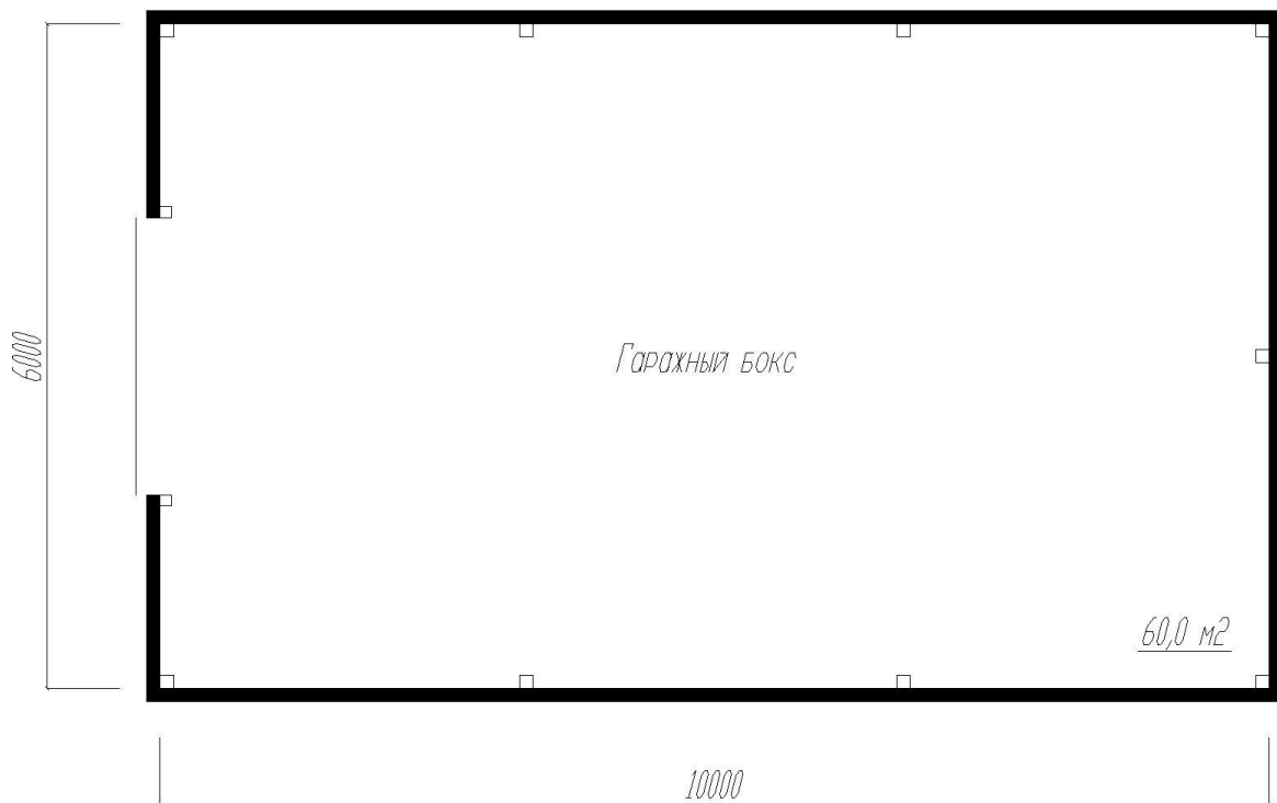
План этажа
